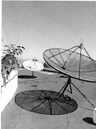
Reorientación de antena al satélite 117 ajuste de azimut e inclinación para recibir señal
