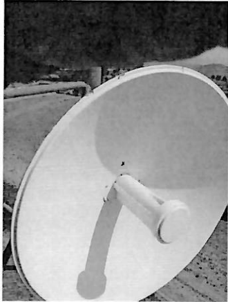
Falla el enlace digital de radio Cambium, se alineo, físicamente y por software, pero no fue posible enlazarlo, se retira para su revisión
